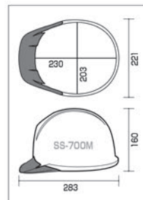
SS-700M 型寸法図
