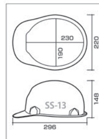
SS-13 型寸法図
