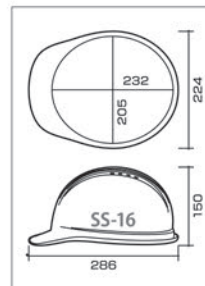
SS-16V 型寸法図
