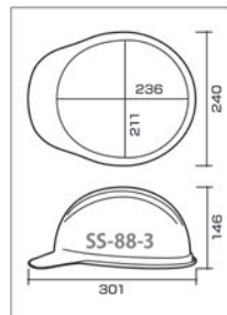
SS-88-3 型寸法図
