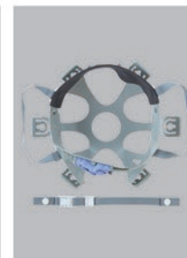
EH 型 - 内装 ・ラチェット式調整 ・耳紐・あご紐付 ▼オープンブライス
