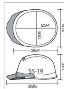
寸法図
