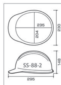
SS-88-2 型寸法図
