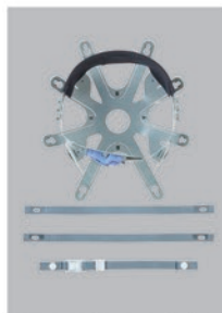
EM-6 型 F-2-O-内装 ・ラチェット式調整 ・耳紐・あご紐付 ¥オープンプライス
